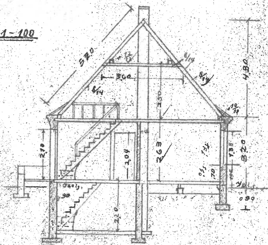
~QUERSCHNITT~
