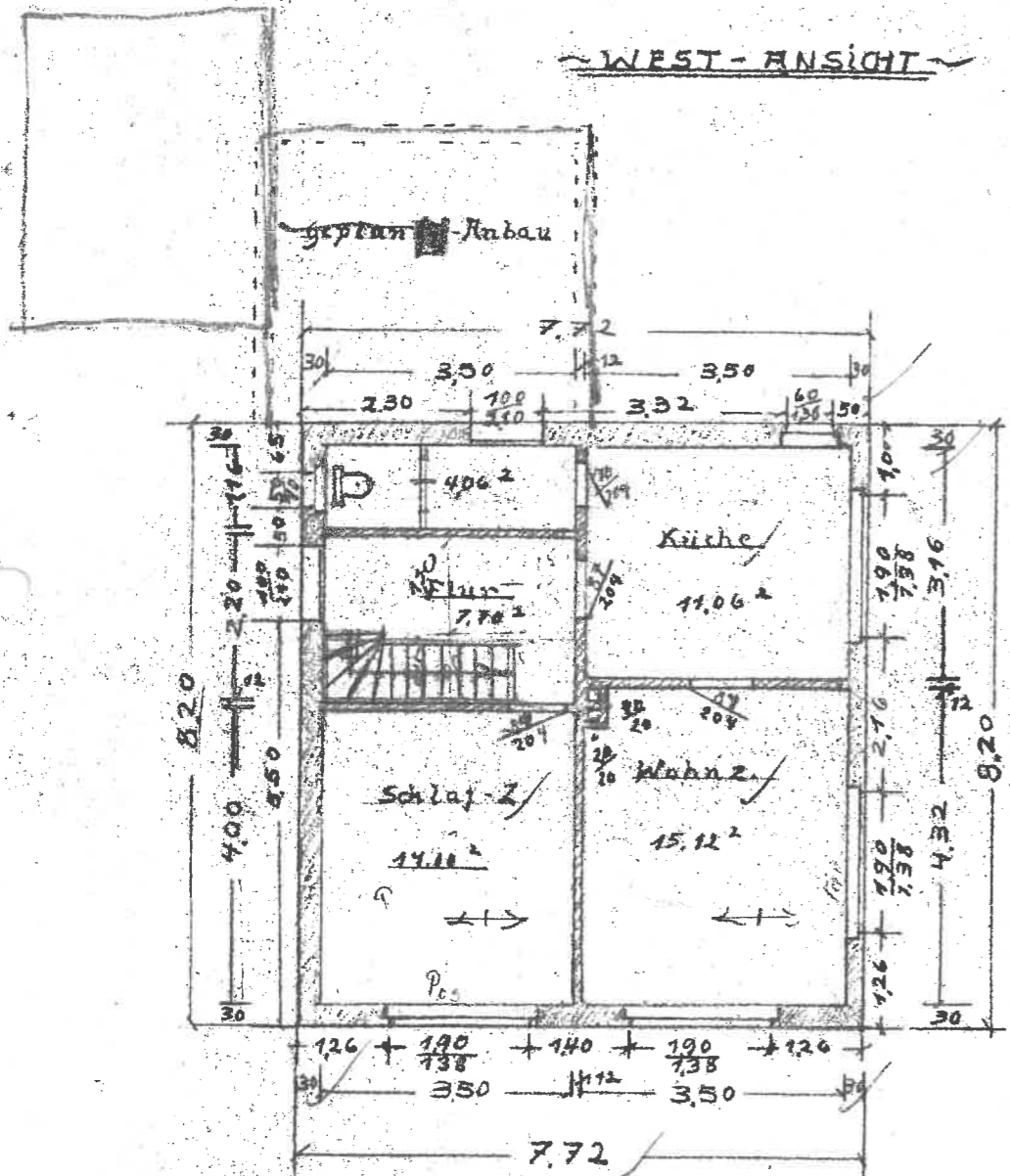
~GRUNDRISS~
