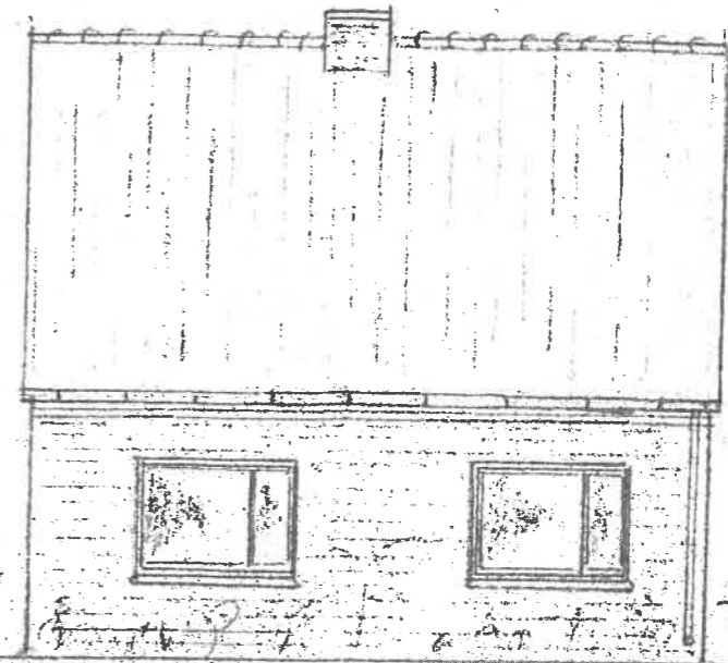
~SÜD-ANSICHT~
