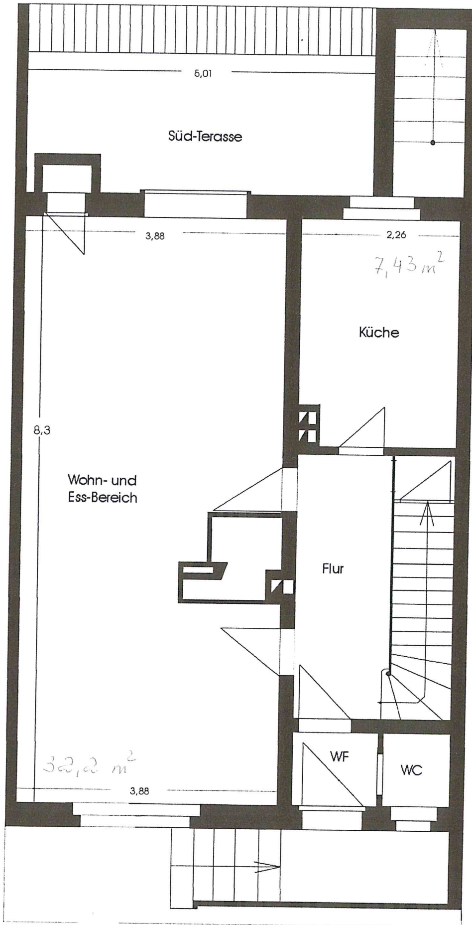
Grundriss Erdgeschoss
