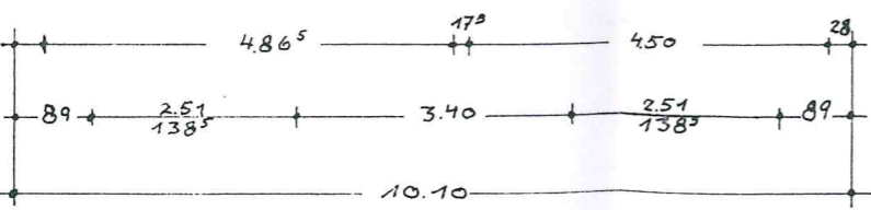
ERDGESCHOSS
